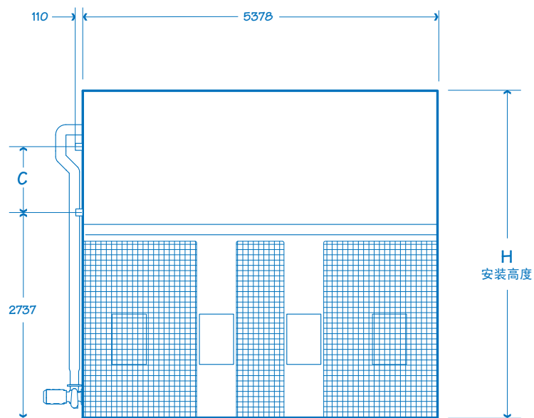
进风口立面图 型号 7055P081 - 7055R121
