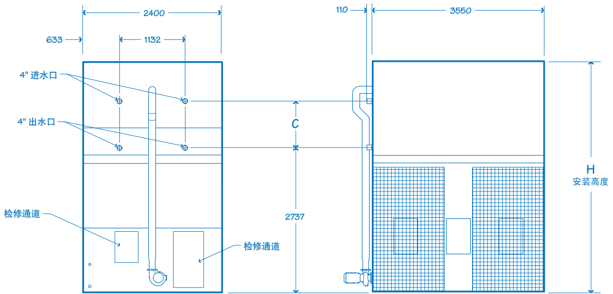
进风口立面图 型号 7054L081 - 7054Q121
